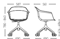
Hollow silent castors Ruedas silenciosas huecas
