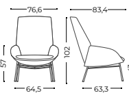
4 Metal legs chair 4 Patas metálicas
