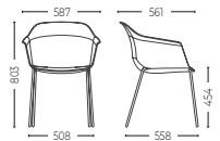
4 metal legs 4 Patas metálicas
